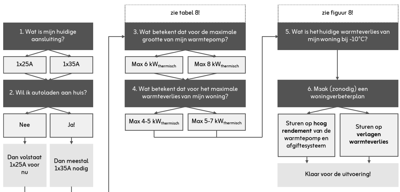
Figuur 9: Stappenplan voor hoe een huishouden binnen een 1-fase aansluiting kan elektrificeren
