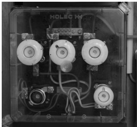
Figuur 2: Een hoofdzekering met transparante verzegelde klep, met daarachter smeltzekeringen. Beeld: Grotius op Klusidee.nl
