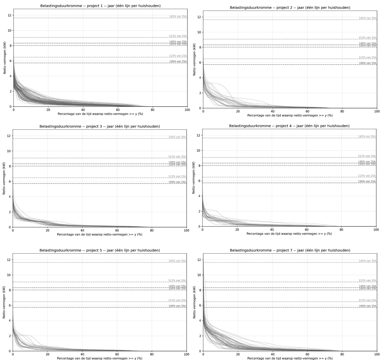
Figuur 10: Jaarbelastingduurkrommes van projecten 1, 2, 3, 4, 5 en 7
